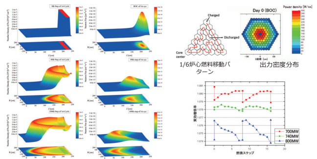
CANDLE燃烧炉の プルトニウム初期炉心 Pu-239、中性子束分布
